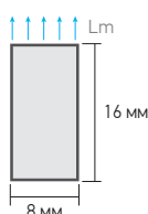
СЕЧЕНИЕ ЛЕНТЫ
